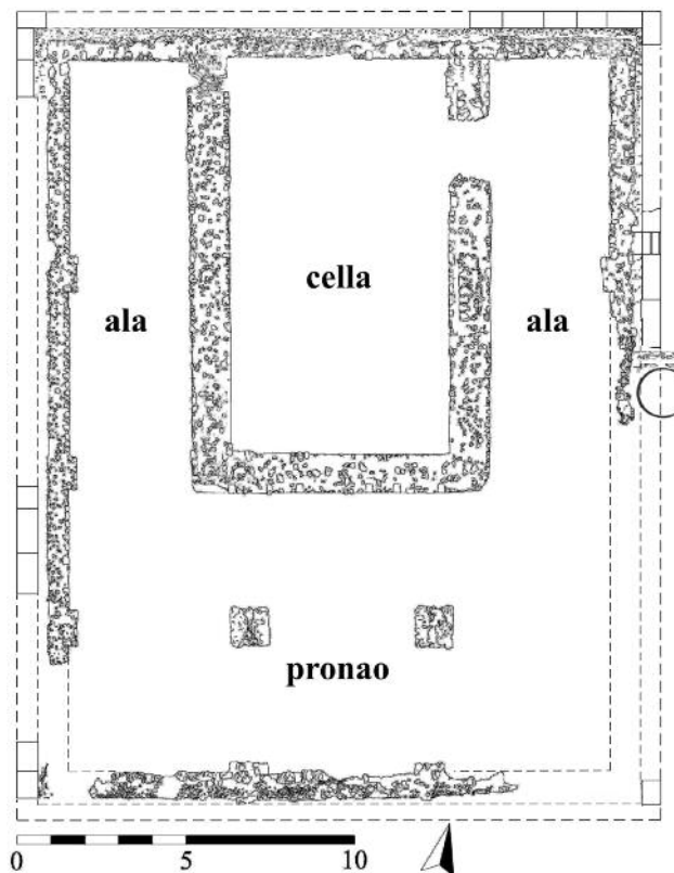
Fig. 3. Fabraeria Nova: resti del tempio maggiore (Tempio A) (aggiornamento 2015 del rilievo SBAL)
